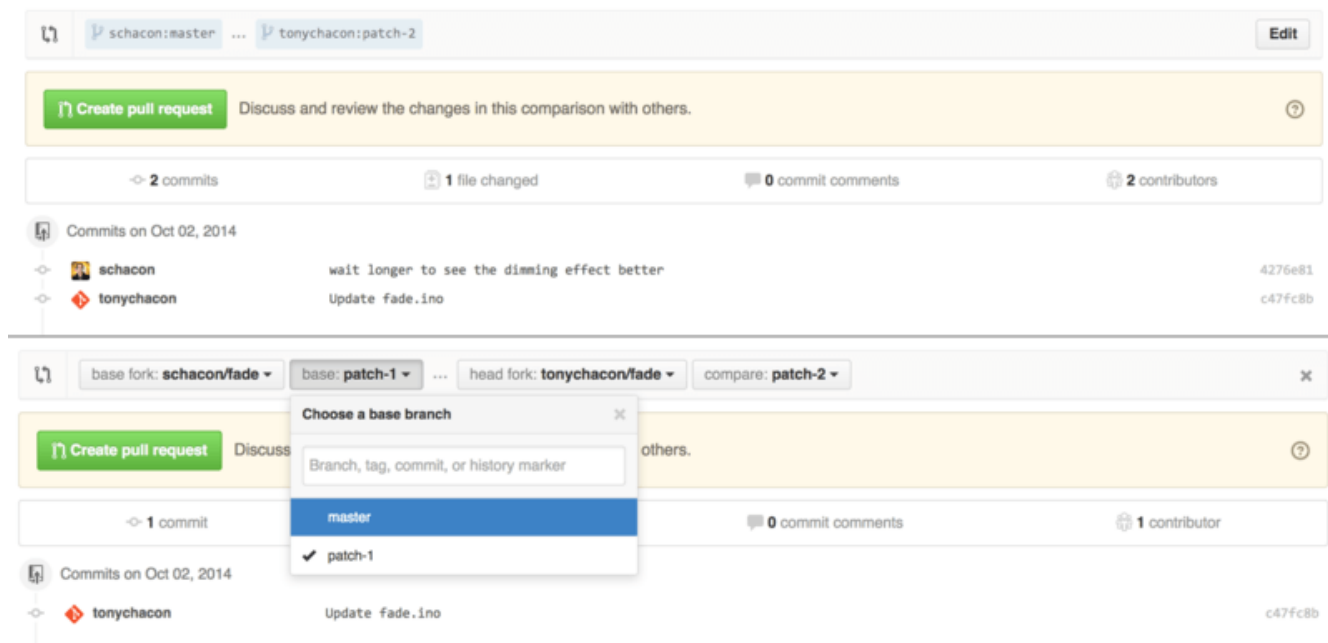
Figure 117. Вручну змінюємо цільову гілку та форк Запиту на Пул.
