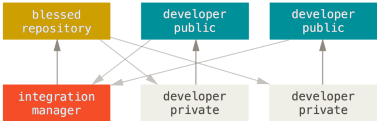
Figure 54. Процес роботи з менеджером інтеграції.
