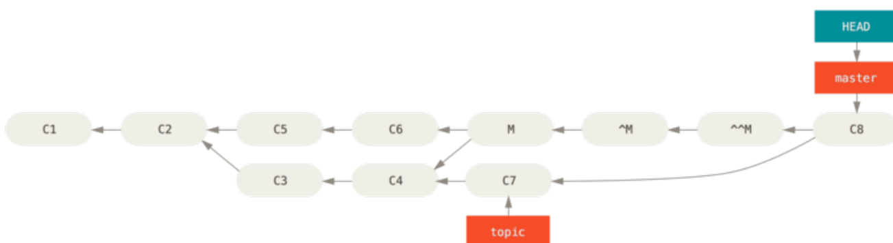
Figure 141. Історія після повторного злиття вивернутого злиття
