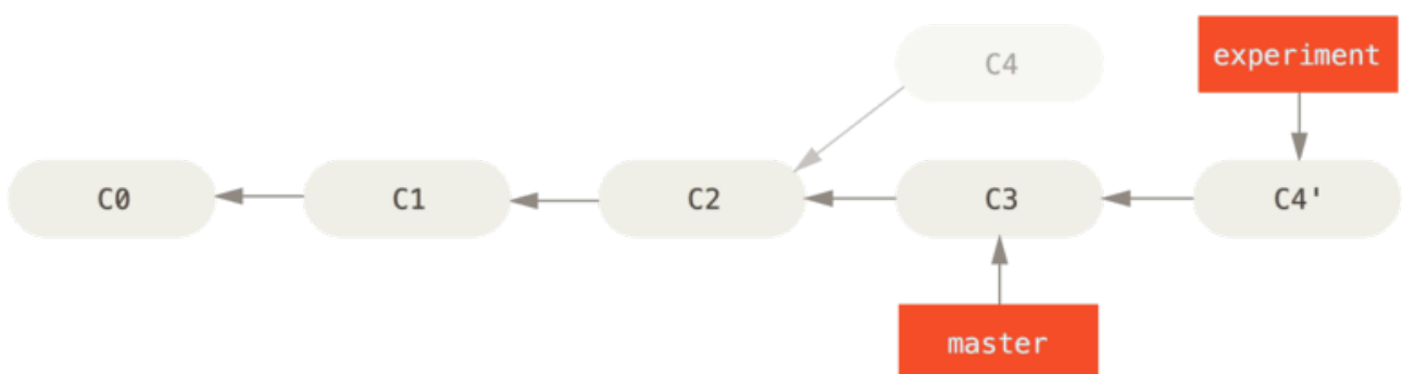
Figure 37. Перебазовування зміни з C4 на C3
