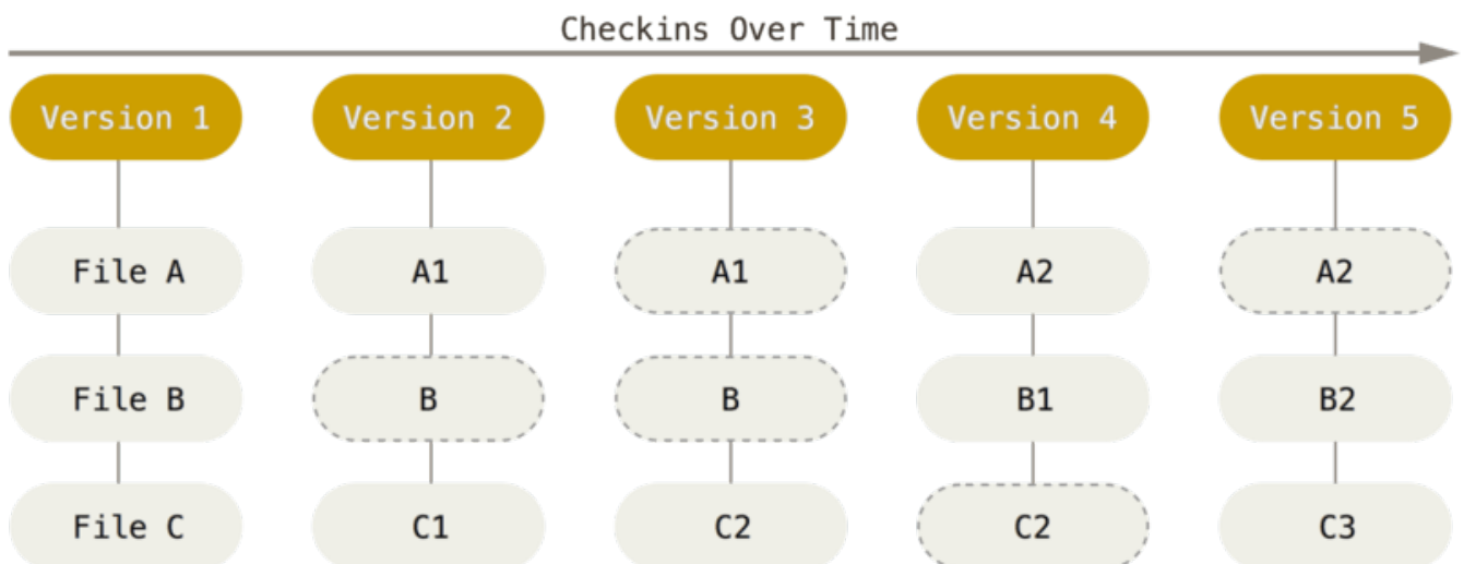
Figure 5. Зберігання даних як знімків проекту за хронологією.
