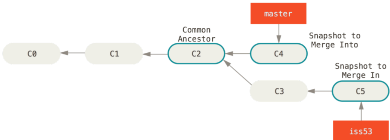
Figure 24. Три відбитки типового злиття
