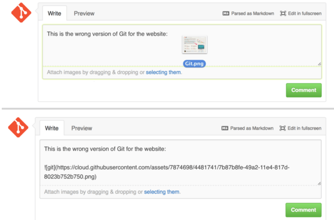
Figure 108. Перетягування зображень щоб відвантажити та автоматично вбудувати їх.
