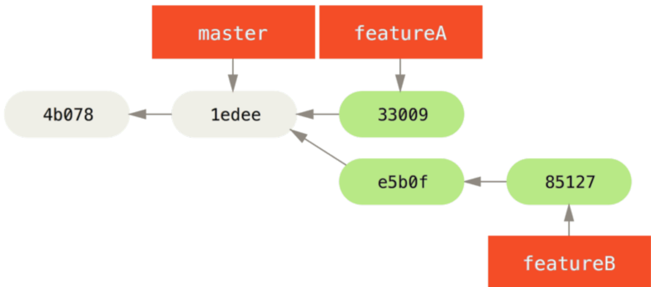
Figure 65. Початкова історія комітів Джесіки.
