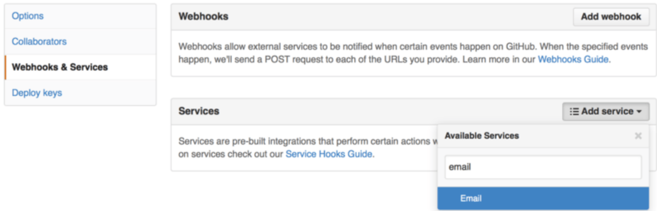
Figure 129. Секція конфігурації Сервіси та Хуки.
